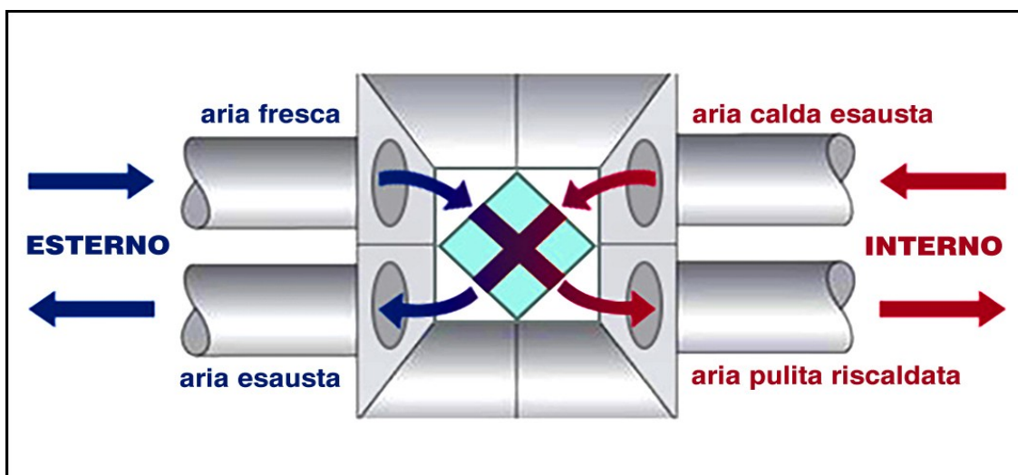
Figura 2: Sistema VMC con filtraggio aria e recupero di calore
