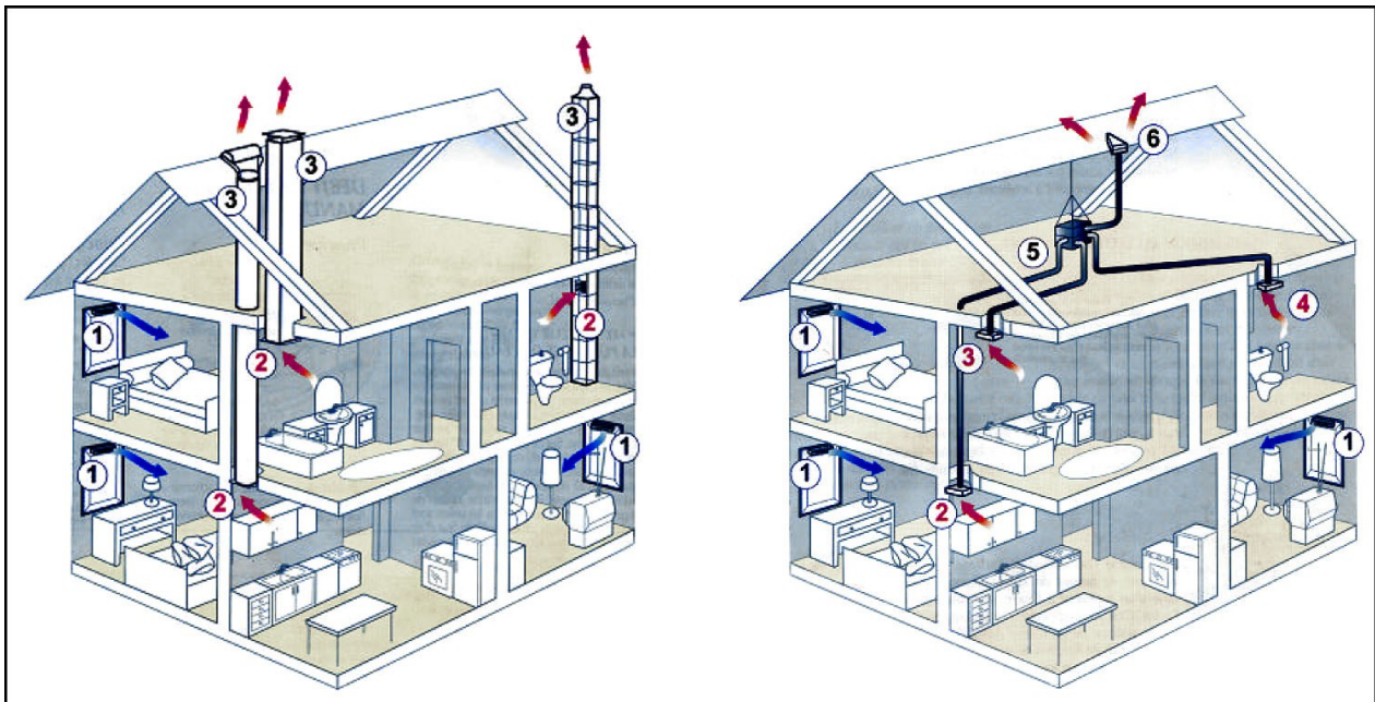
Figura 1: A sx sistema di ventilazione tradizionale - A dx Sistema di ventilazione meccanica controllata
